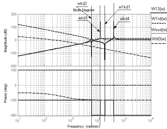
Рис.1. Логарифмические амплитудные и частотные характеристики объекта управления контура давления W_{13}(\omega) , регулятора давления W'_{rd}(\omega) , внутренней отрицательной обратной связи в гидросистеме W_{osd}(\omega) разомкнутого контура активного тока W_{rt0}(\omega) без учета сил диссипации
