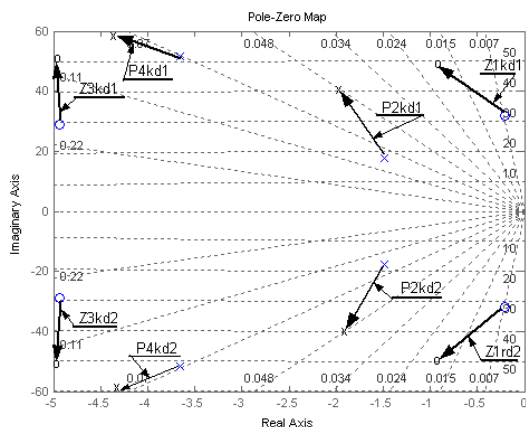
Рис.2. Перемещения нулей ( Z_{1kd1} , Z_{1kd2} , Z_{3kd1} , Z_{3kd2} ) и полюсов ( P_{1kd1} , P_{1kd2} , P_{3kd1} , P_{3kd2} ) на комплексной плоскости динамического звена W_{\ddot{a}}(p) , обусловленное податливостью гидросистемы и канатно-полиспастовой системы в зависимости от жесткости каната и веса става
